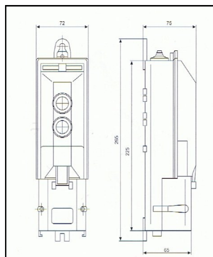
Kabelaflastning i top med PG forskruring.
