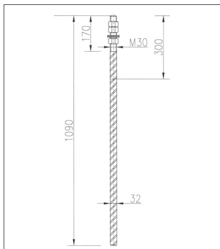
M30 x 1090 mm bolt. Galvaniseret topdel, skiver og møtrikker
