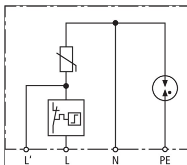
Principdiagram DCOR L 2P SN1860. Varistor mellem fase/nul. Gnistgab mellem nul/PE.
