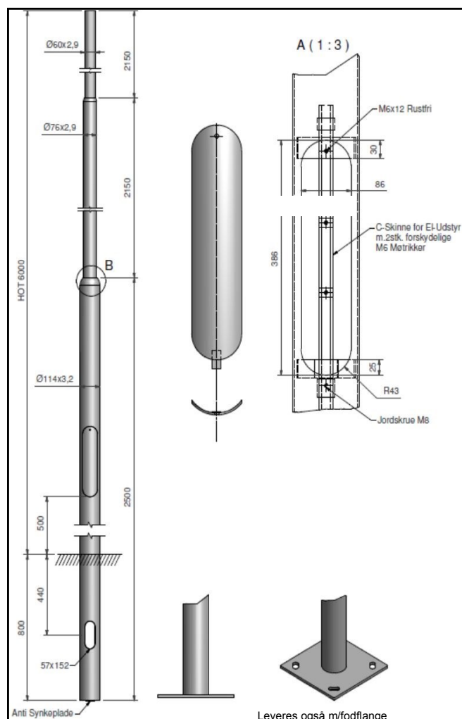
Kraftig parkstolpe LPH = 6,0m m/indfældet luge, Ø 60 mm top
